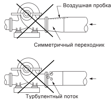
Рис. 27 Переходники, из-за которых образуются воздушные пробки и турбулентность
