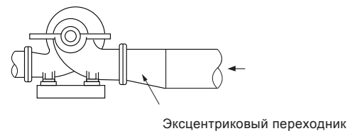
Рис. 26 Правильно смонтированный переходник
