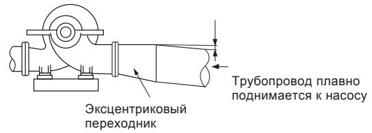
Рис. 29 Правильно смонтированный всасывающий трубопровод
