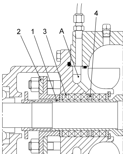
Рис. 19 Вид в разрезе сальника с внутренней промывочной жидкостью
